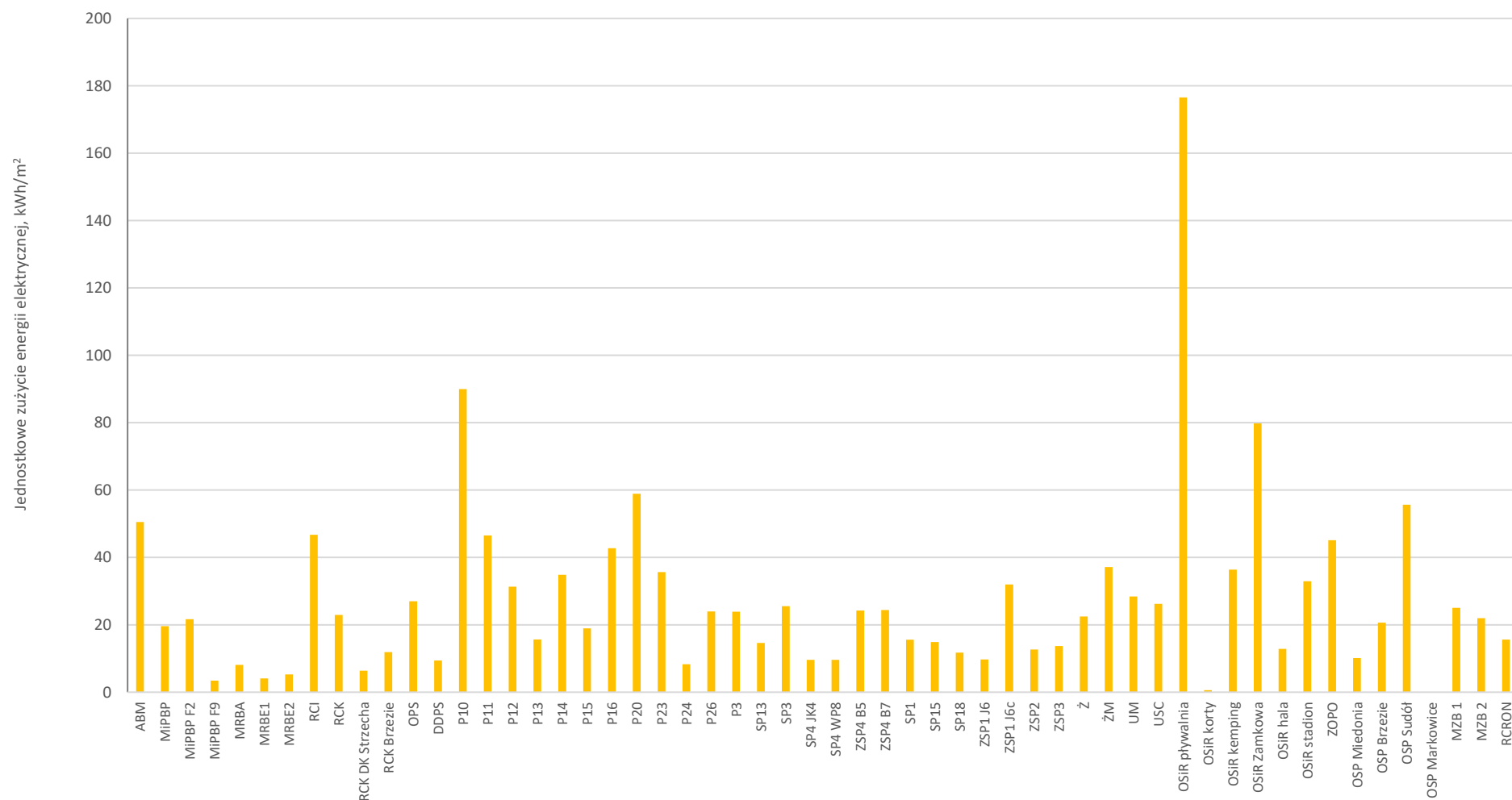
Rysunek 6.2 Jednostkowe zużycie energii elektrycznej w odniesieniu do powierzchni użytkowej dla analizowanej grupy obiektów
