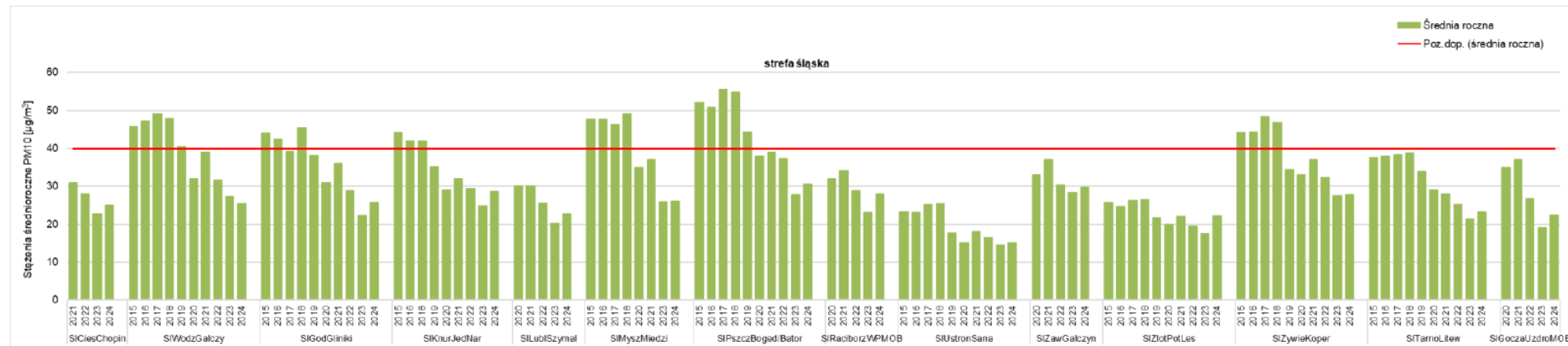
Rysunek 3.8. Średnie roczne stężenia pyłu PM10 w strefie śląskiej w latach 2015-2024
