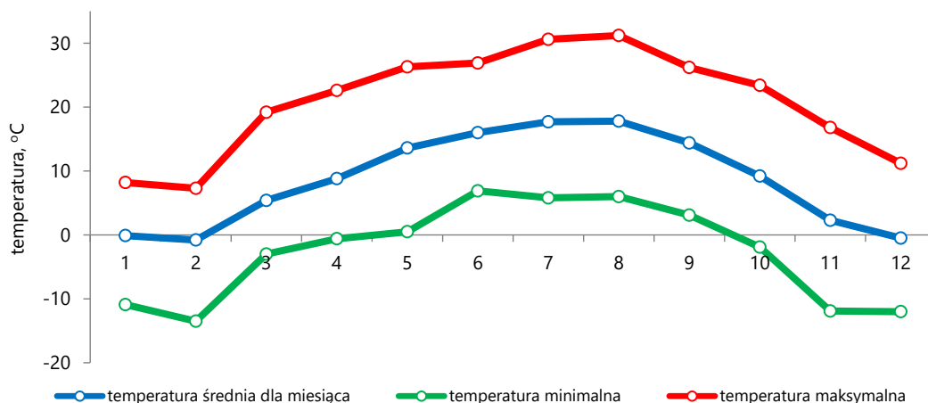
Wykres 2.1 Średnie wieloletnie dane temperaturowe dla stacji meteorologicznej - Racibórz Studzienna
