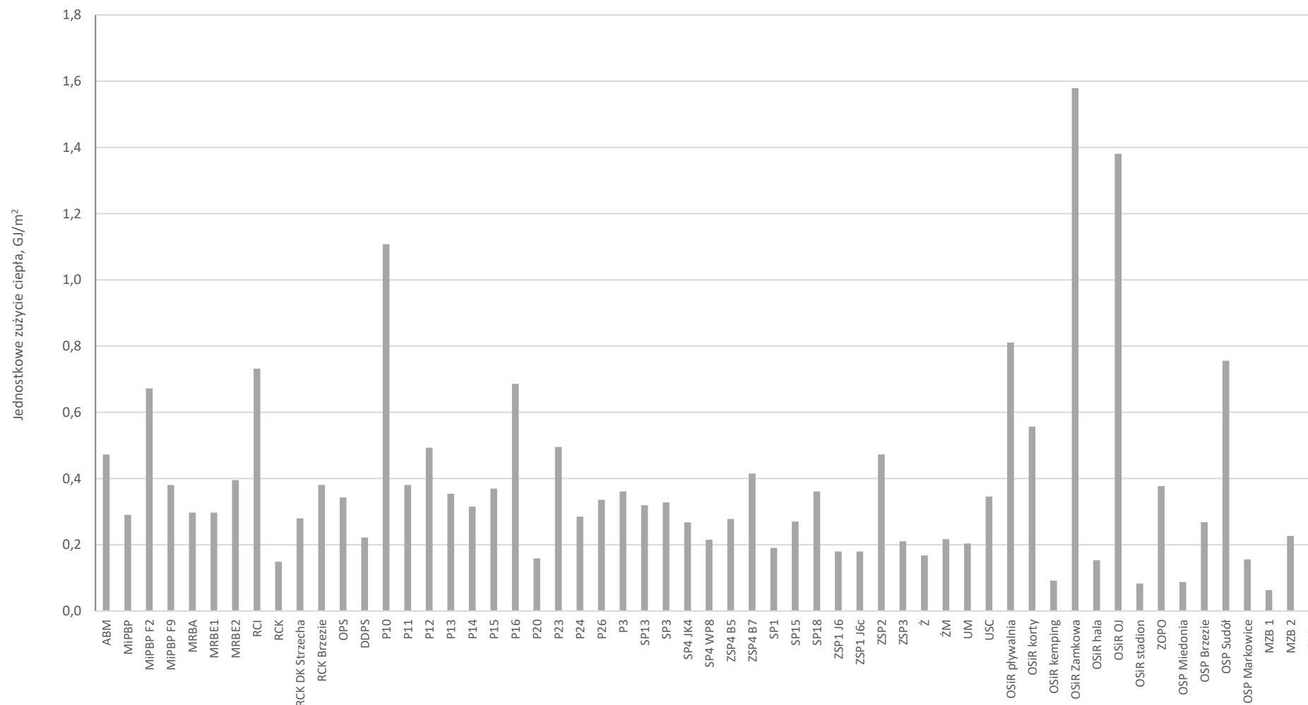
Rysunek 6.1 Jednostkowe wskaźniki zużycia energii do celów grzewczych dla analizowanej grupy obiektów
